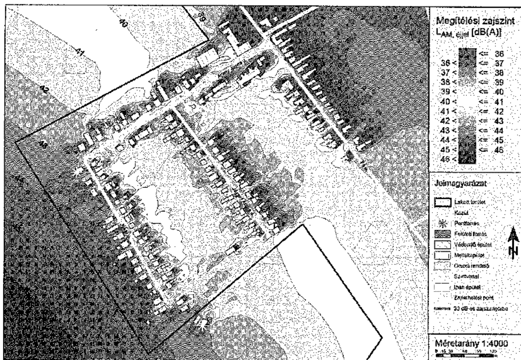
4-8. ábra Zajkibocsátási zajterkép (részletes - Iváncsa, Jókai u. és környéke)
